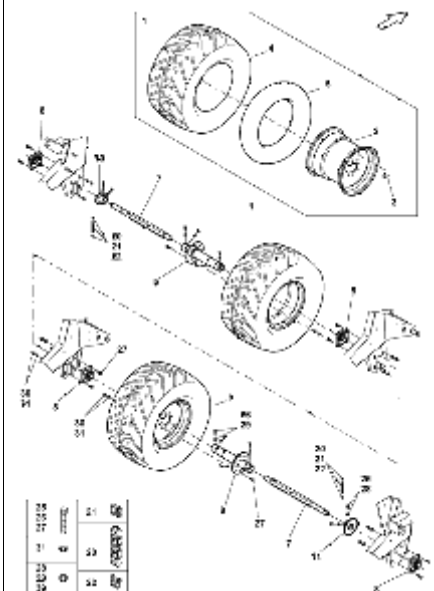
C4 Terra-Bereifung 31x15,5/15 -- ED 601 Seite 68
